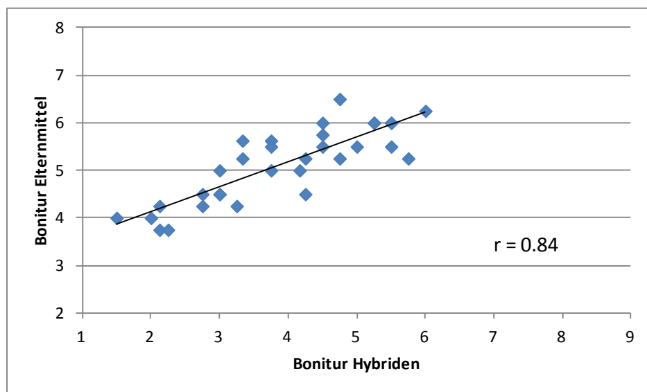
Abb. 3: Zusammenhang zwischen Helminthosporium Blattfleckenbonitur von 32 mittelfrühen xperimentalhybriden, getestet über 2 Jahre in Süddeutschland und dem Elternmittel aus der Linieneigenleistung (Bonitur von 1 bis 9; 1 = resistent, 9 = hochanfällig)
