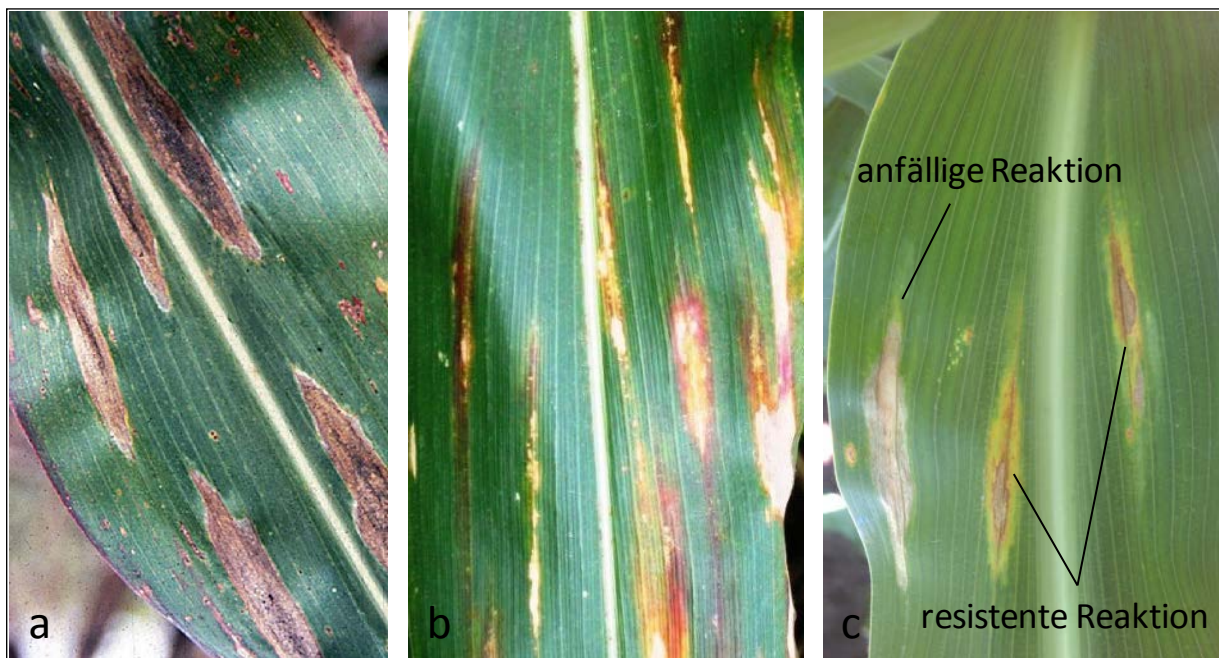
Abb.2: Blattfleckenausprägung als Reaktion auf Setosphaeria turcica Rassen bei Pflanzen mit und ohne Ht1 Resistenz (a = anfällige Reaktion ohne Ht1 ; b = resistente Reaktion von Ht1 bei Infektion mit Rasse 0; c = anfällige und resistente Reaktion von Ht1 bei Infektion mit Rasse 0 und 1)
