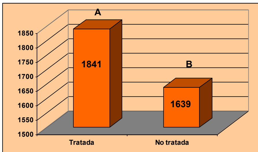
Figura 10. Prueba de Tukey para la variable rendimiento con respecto al tratamiento. Letras diferentes expresan diferencias significativas a nivel de p \leq 0,05
