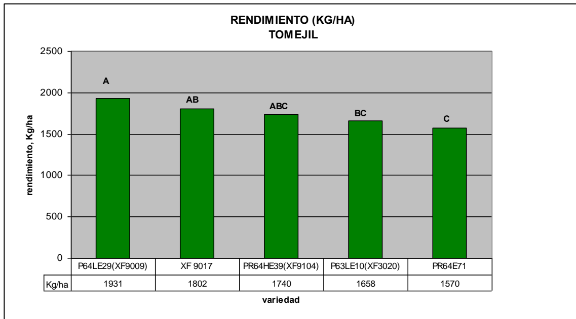
Figura 9. Prueba de Tukey para la variable del rendimiento grano con respecto a la variedad. Letras diferentes expresan diferencias significativas a nivel de p \leq 0,05
