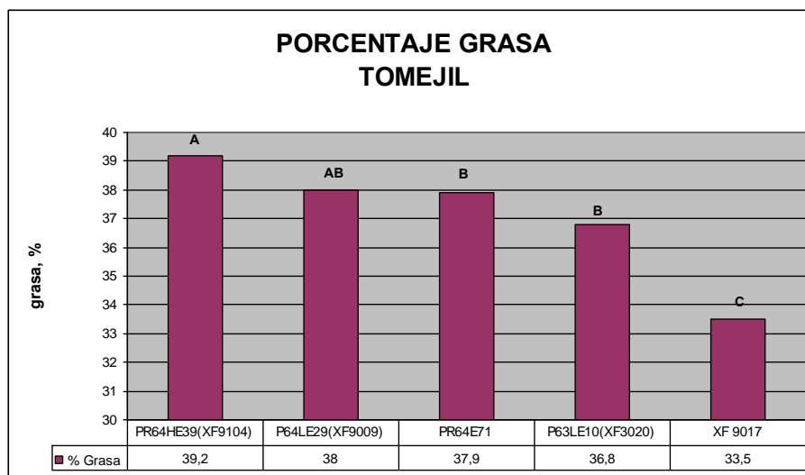
Figura 11. Prueba de Tukey para la variable % grasa con respecto a la variedad. Letras diferentes expresan diferencias significativas a nivel de p \leq 0,05
